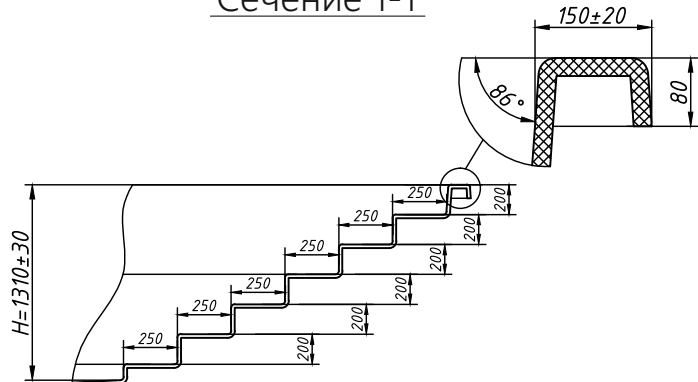
Сечение 1-1
